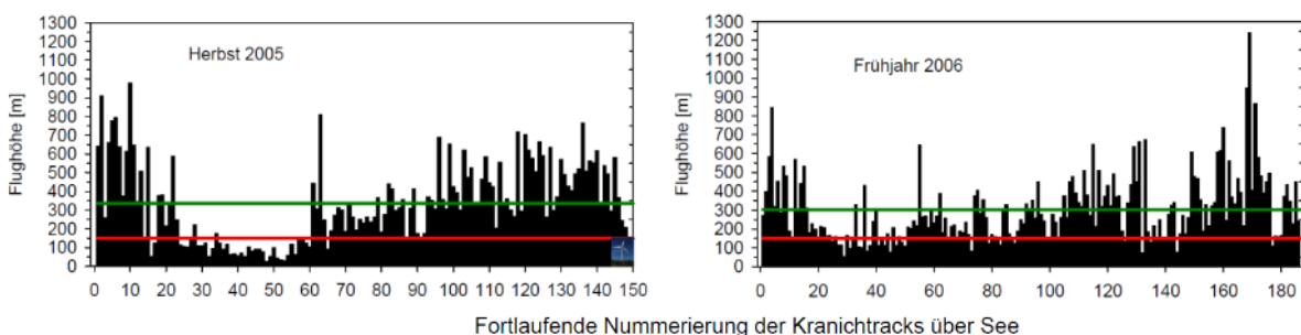
Ilustracja 49: Wysokość lotu nad poziomem morza podczas jesiennej i wiosennej wędrówki żurawi (zielona linia: średnia wysokość przelotu w całym sezonie; czerwona linia: maks. wysokość turbin wiatrowych; BELLEBAUM et al. 2008).
