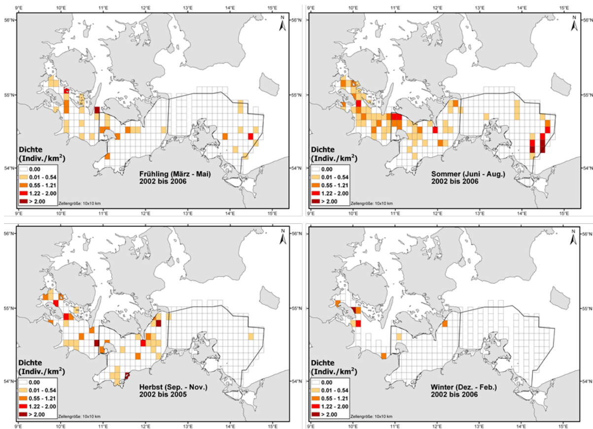
Ilustracja 37: Sezonowy wzór rozmieszczenia morświnów w południowo-zachodniej części Morza Bałtyckiego (2002-2006). Mapy rastrowe są pozbawione nakładów. Pokazane jest średnie zagęszczenie morświnów na komórkę siatki (10x10km) a) wiosną (marzec-maj), b) latem (czerwiec-sierpień), c) jesienią (wrzesień-listopad) i d) zimą (grudzień-luty, źródło: GILLES i in. 2007, s.126 i nast.).
