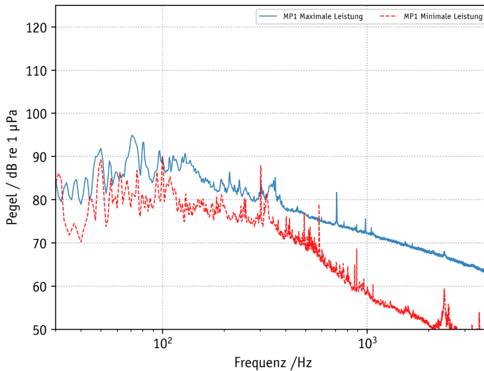
Abbildung 17: Beispielhafte Gegenüberstellung der Schmalband-FFT-Spektren für eine ausgewählte Windanlage mit und ohne Getriebe aus Abbildung 16 in den Windklassen „niedrig“ (Anlagen im Stillstand) und Windklasse „hoch“ (Anlagen unter Nennleistung).
