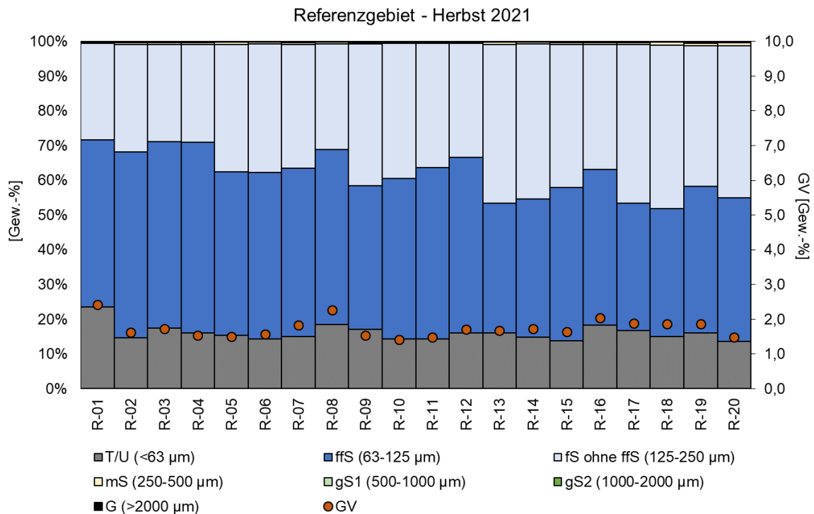
Abb. 47: Korngrößenanteile und Glühverluste der Sedimente im Referenzgebiet (R) im Herbst 2021 auf Stationsebene (Mittelwert aus drei Greifern/Station).
