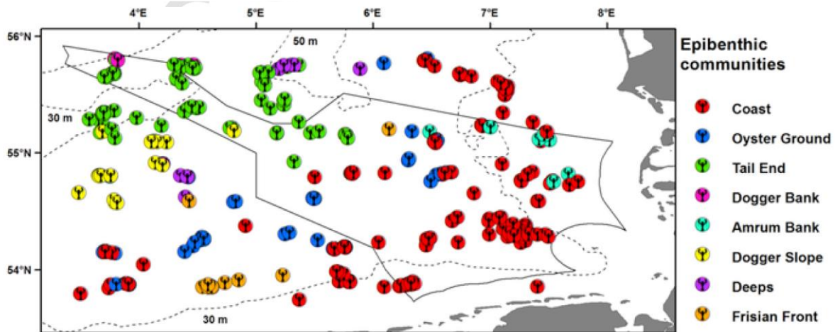
Abb. 80: Verteilung der acht auf Basis von Clusteranalysen identifizierten Epibenthos-Gemeinschaften. Abbildung aus NEUMANN et al. (2017).
