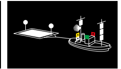
Schleppverbände in Fahrt; Links: bis 200 m Schlepplänge (Schlepper nicht über 50 m Länge); Mitte: mit längsseits geschleppten Anhängen; Rechts: über 200 m Länge, mit außergewöhnlichem Schwimmkörper (schleppendes Fahrzeug über 50 m lang)
